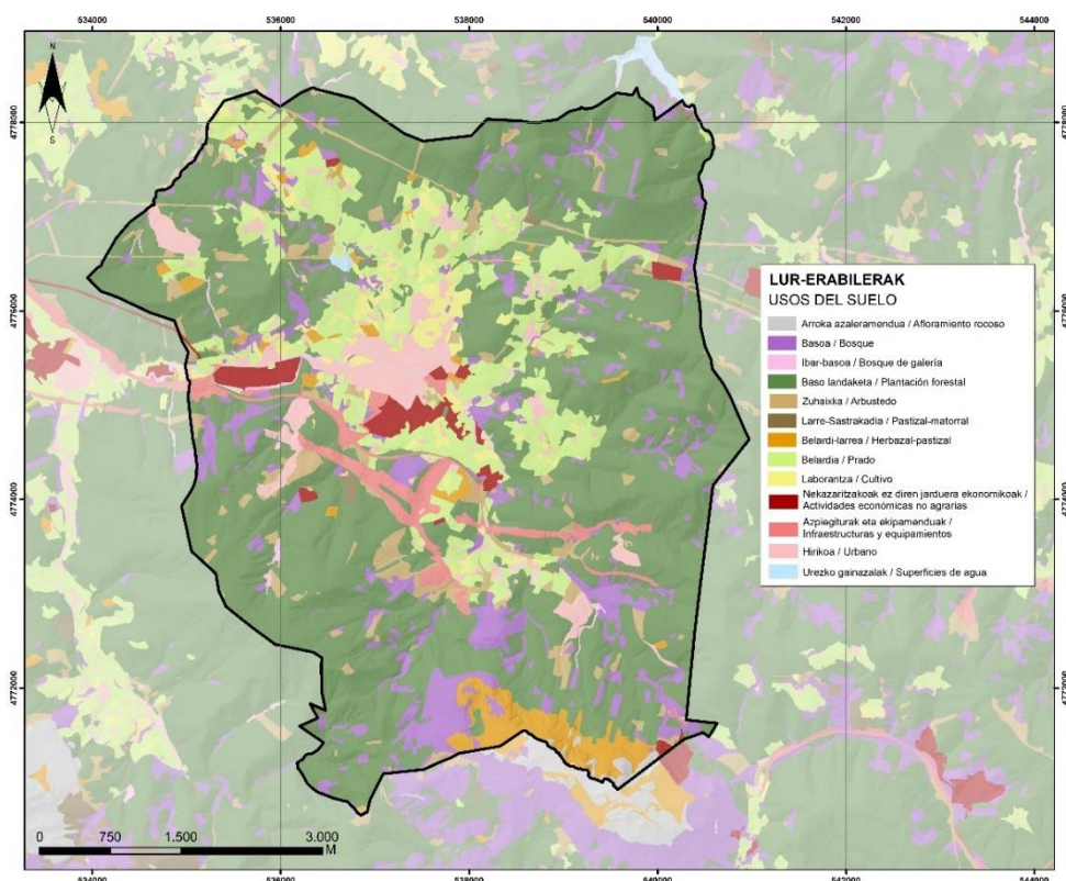
15. Irudia. Lurzoruaren erabilerak Elorriko udalerrian. Iturria: geoEuskadi.
