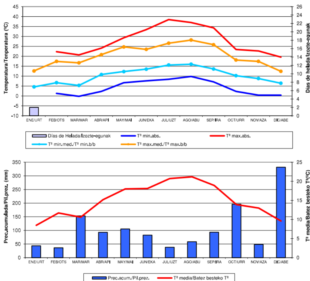
9. Irudia. 2024. urteko diagrama ombrotermikoa eta klimograma, Elorrioko estazio meteorologikorako.
