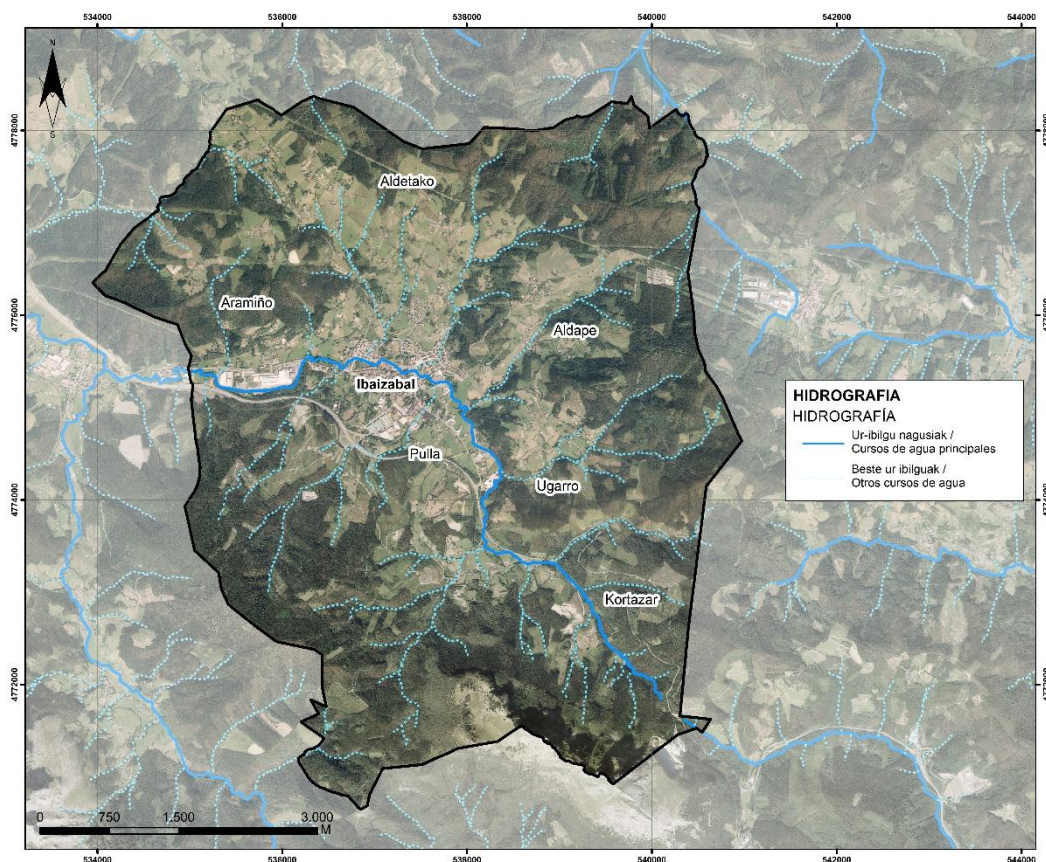
17. Irudia. Elorrioko udalerriko sare hidrografikoa. Iturria: geoEuskadi.
