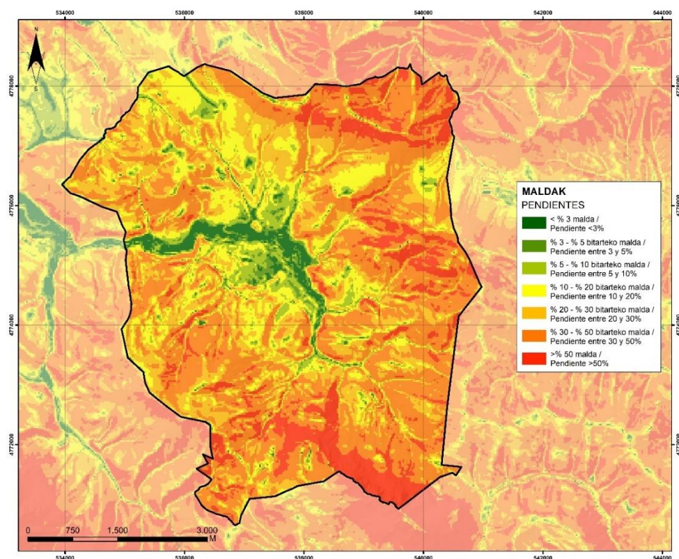
13. Irudia. Elorriko udalerriko malden inklinazioa. Iturria: geoEuskadi.
