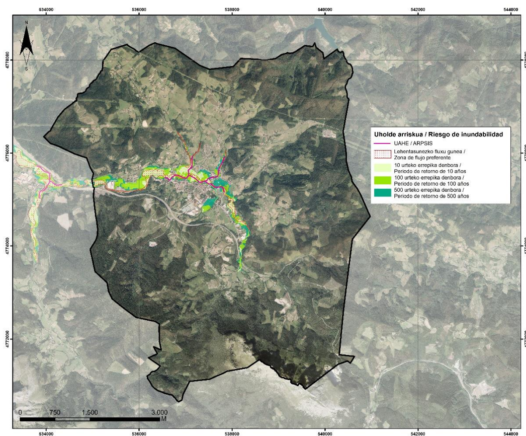
18. Irudia. Uholde-arriskua errepikatze-denboren arabera (10, 100 eta 500 urte). Iturria: geoEuskadi.
